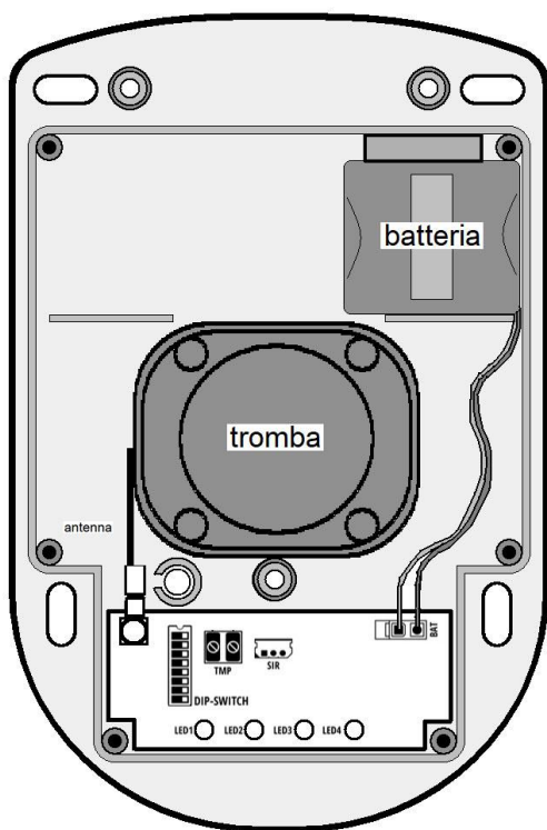
Figura 1 – Identificazione delle parti
