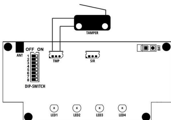
Figura 2 – Scheda elettronica
